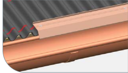
Aluminyum Saçak Çıtası
